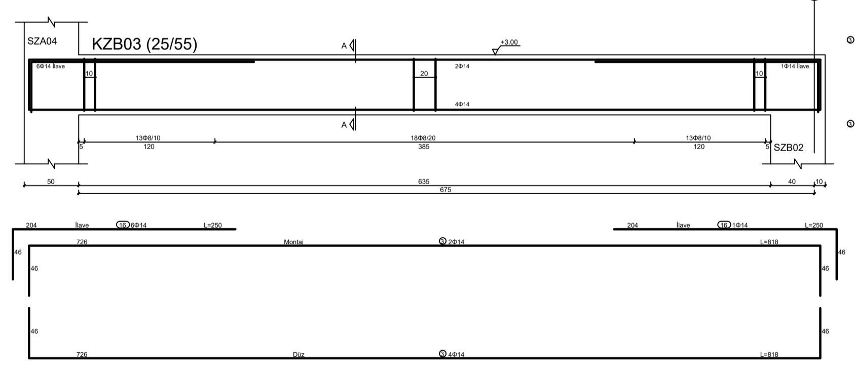
ZEMİN KAT KİRİŞ DONATI AÇILIM DETAYI ÖLÇEK: 1/20
