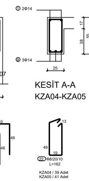
ZEMİN KAT KİRİŞ DONATI AÇILIM DETAYI ÖLÇEK: 1/20
